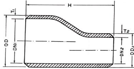
Redução excêntrica nº 1105.
