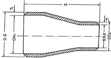
Redução concêntrica nº 1104.
